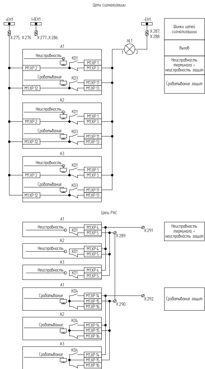
Рисунок В.11 – Схема электрическая принципиальная (часть 11)
