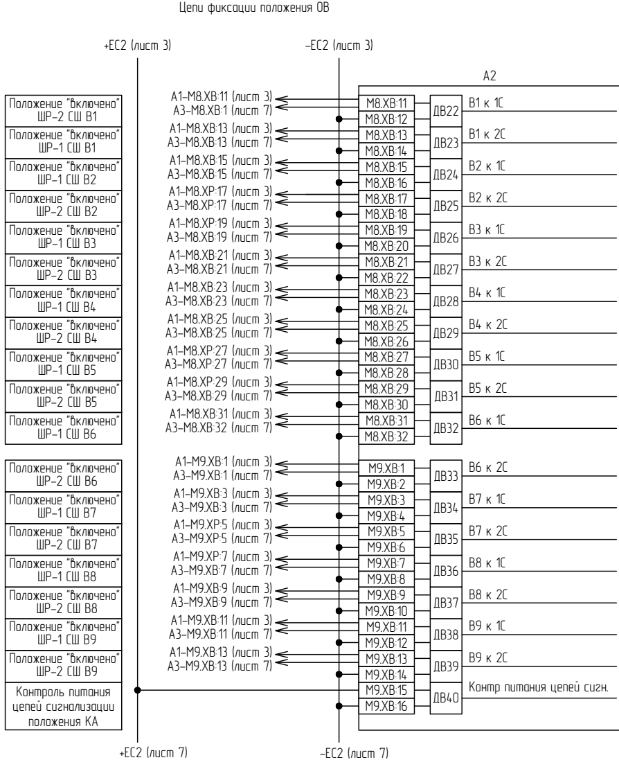
Рисунок В.5 – Схема электрическая принципиальная (часть 5)
