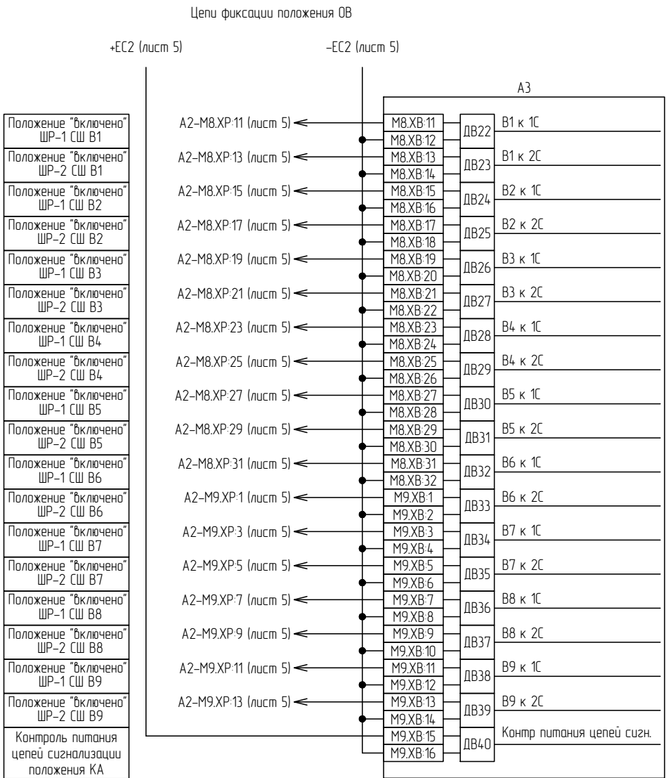
Рисунок В.7 – Схема электрическая принципиальная (часть 7)
